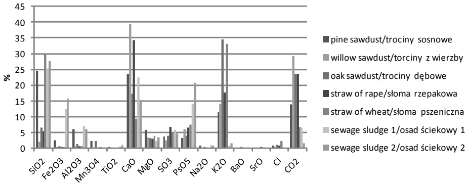
Fig. 4. Ash chemical analysis of analysed feedstock Rys. 4. Chemiczna analiza popiołu
