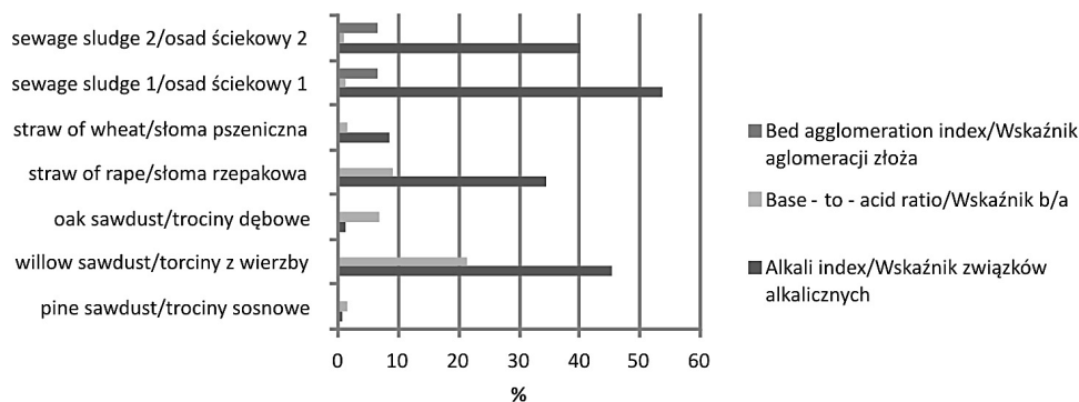
Fig. 5. Slagging/fouling indexes of analysed feedstock Rys. 5. Wskaźniki charakterystyczne dla popiołu
